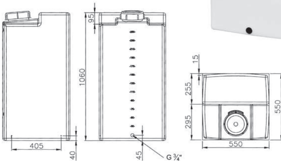
Dosierbehälter BD-A 250
