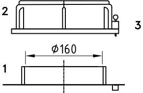
1: Behälteröffnung 2: Schraubdeckel CPF-210 3: Steckschloß
